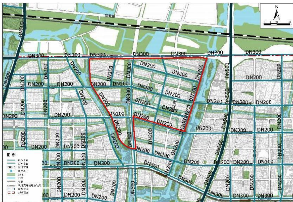
图 3 片区供水管网规划图
