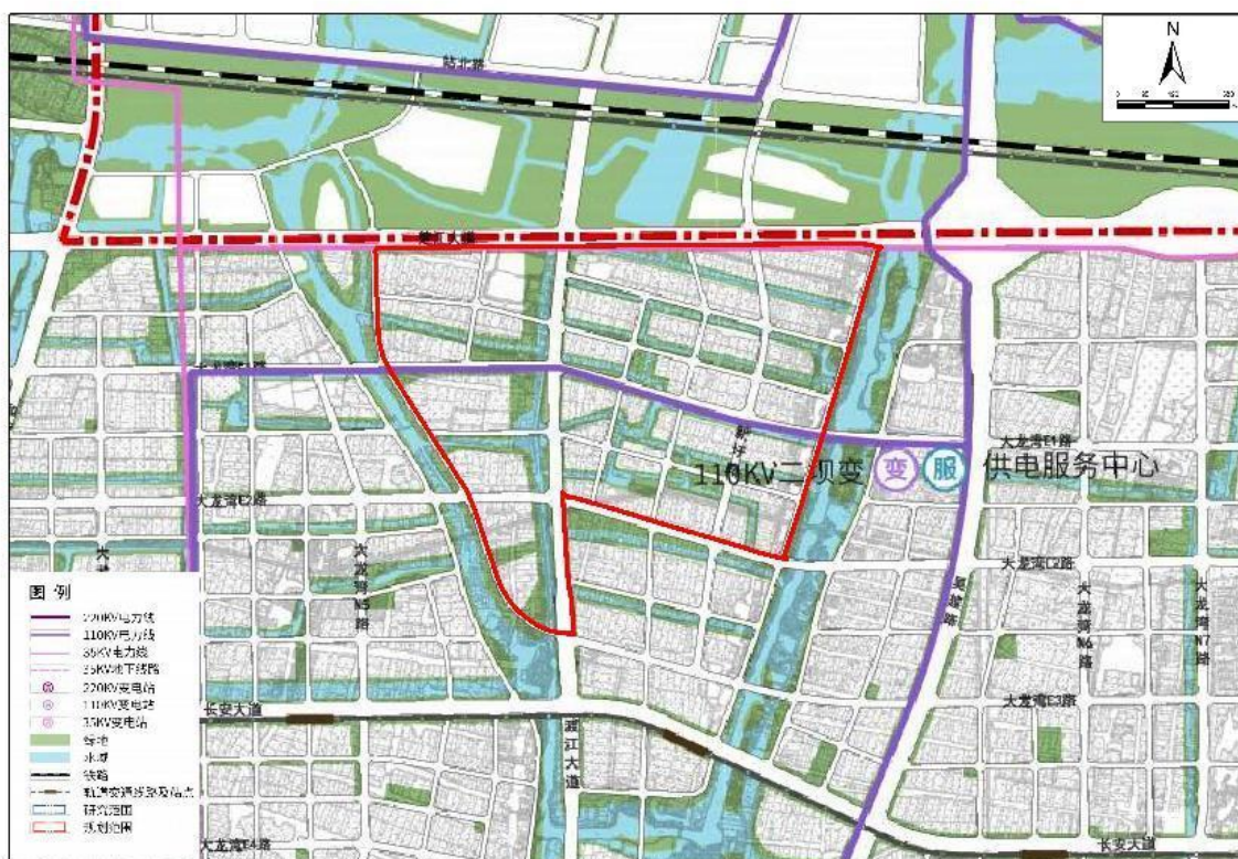
图 5 片区供电设施规划图
