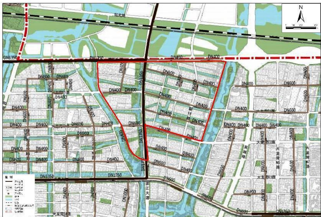
图 4 片区排水管网规划图
